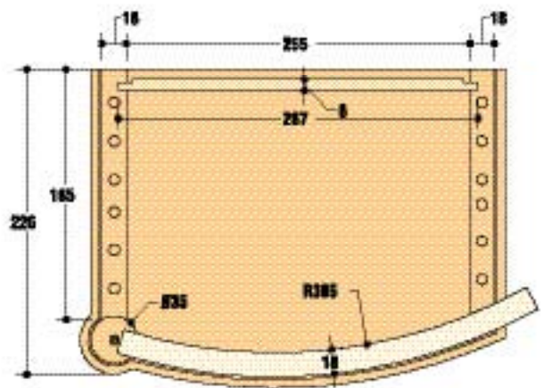
PLAN 1:6
